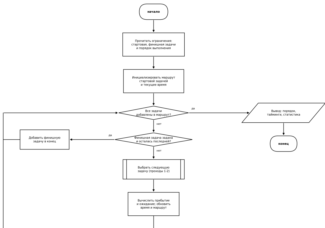
Рисунок Б.1 – Блок-схема алгоритма NNH-TW: основной цикл построения маршрута
